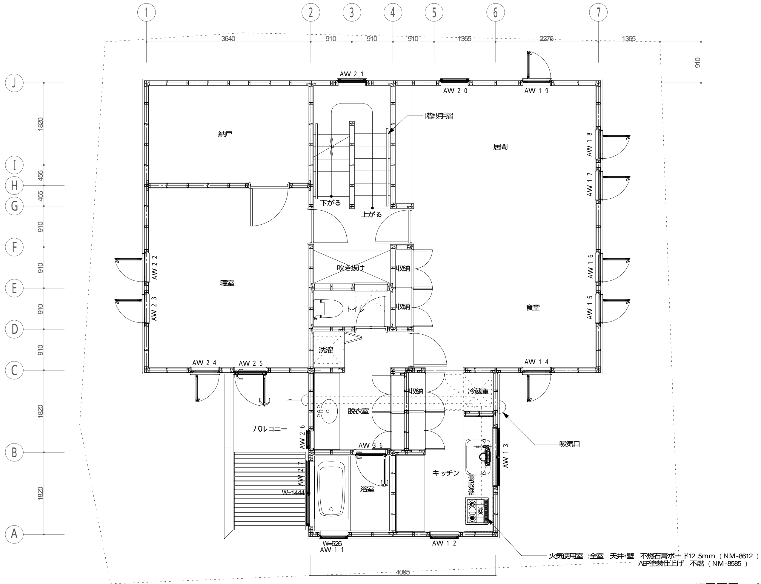
2F平面図 S,1:50
